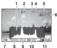
Histogramme luminosité
