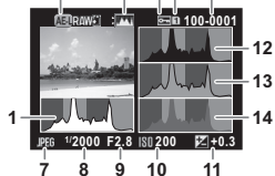
Histogramme RGB
